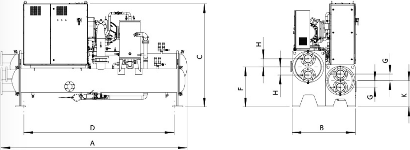
SMP系列冷水机组外形及接管尺寸
